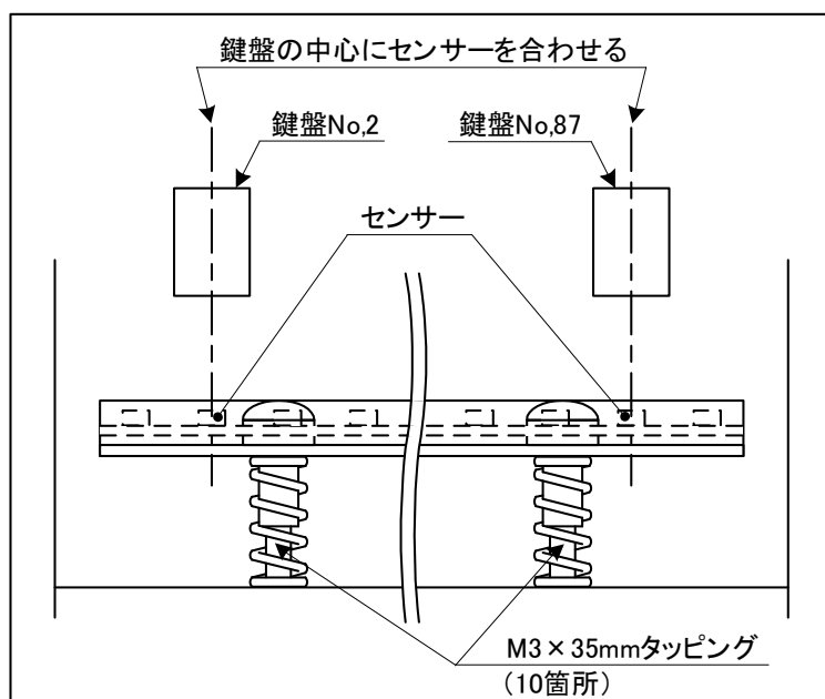
図4.4-4 鍵盤センサー左右位置決め
