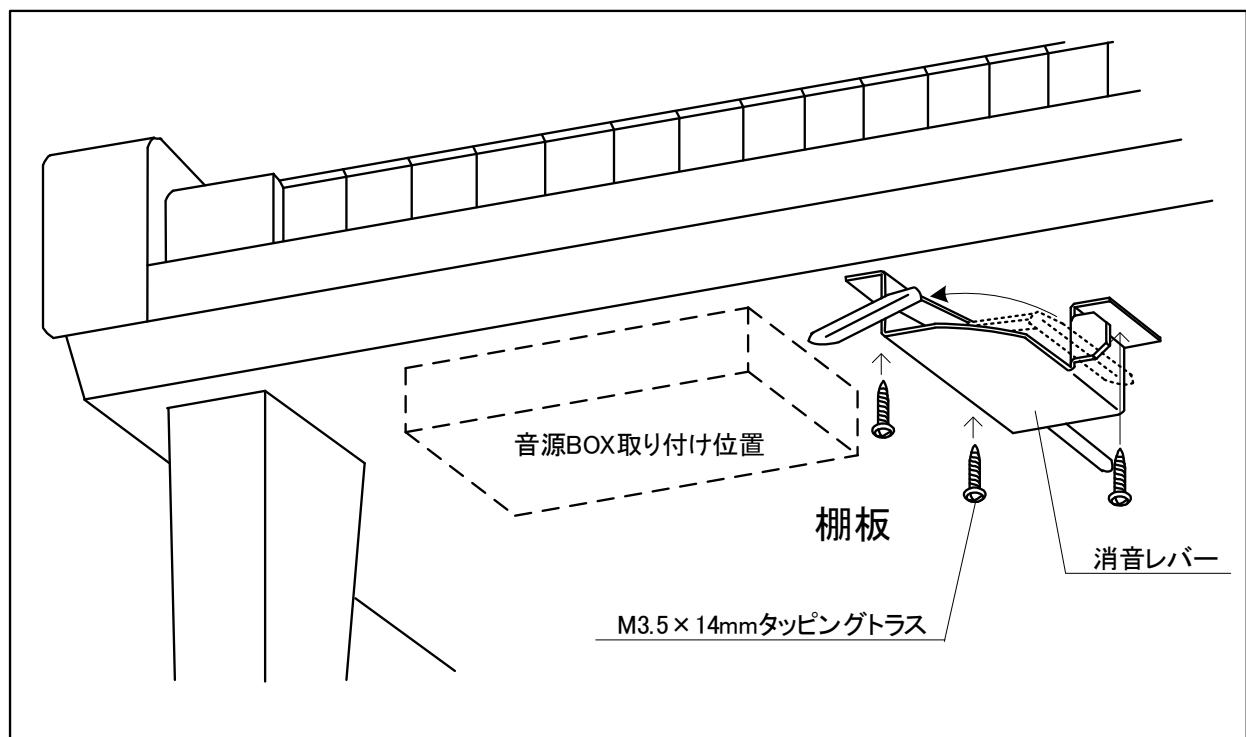
図 4. 6 - 2 消音レバー取り付け位置
