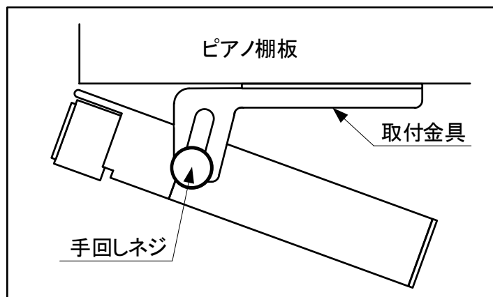
図 4. 7 - 3 音源BOXの角度調整
