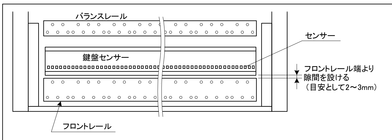
図 4. 4 - 3 鍵盤センサーの取り付け
