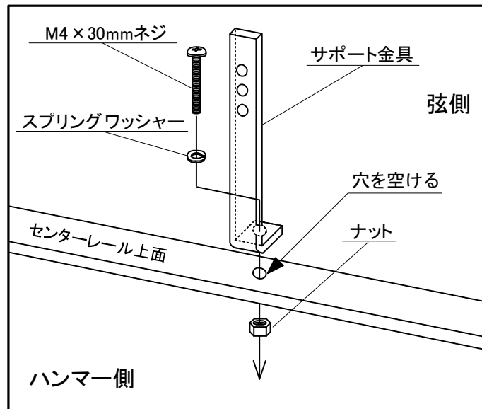
図 4. 3 - 1 サポート金具の取り付け
