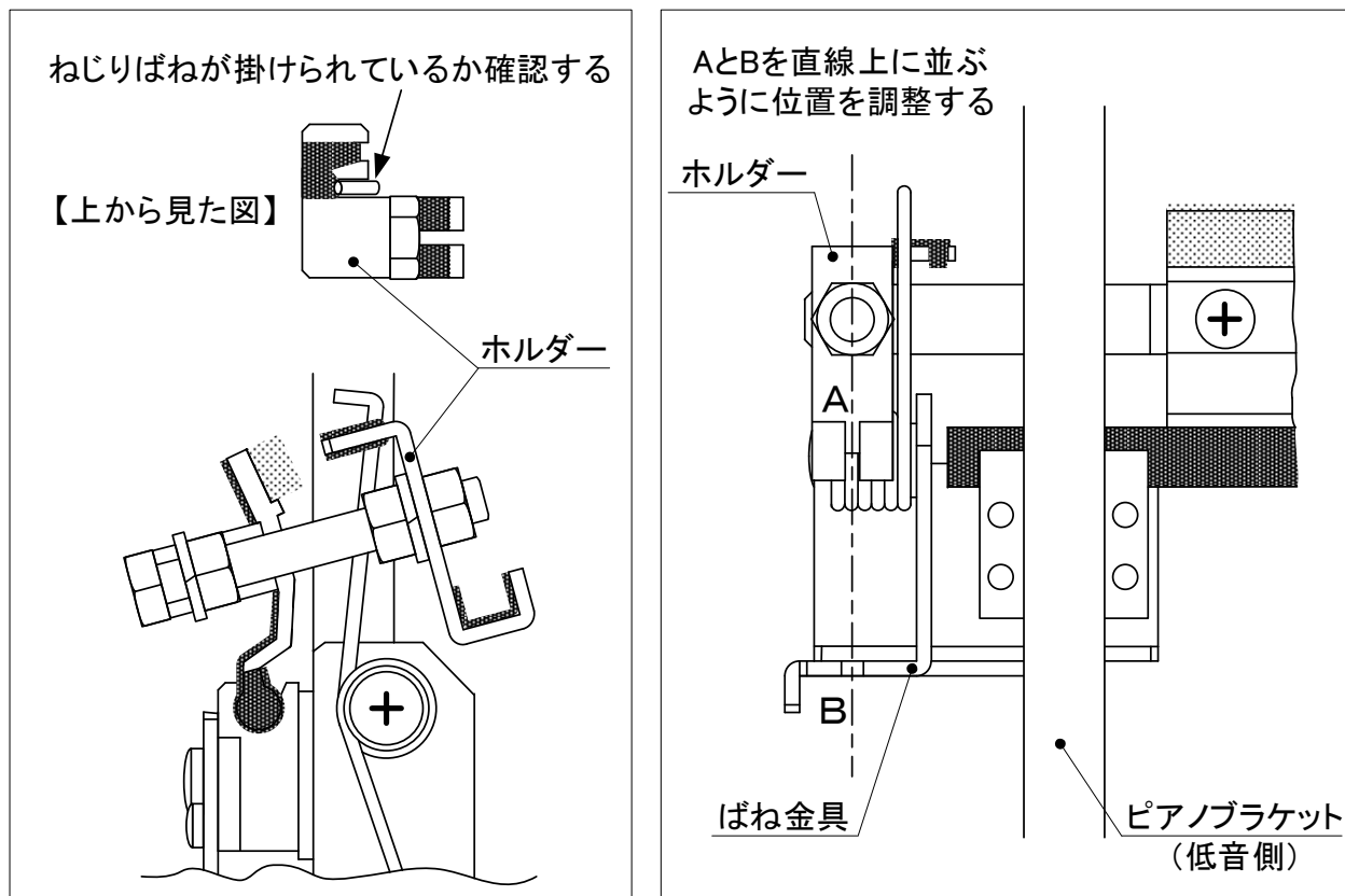
図 4. 3 - 8 ばね掛けと金具の位置調整
