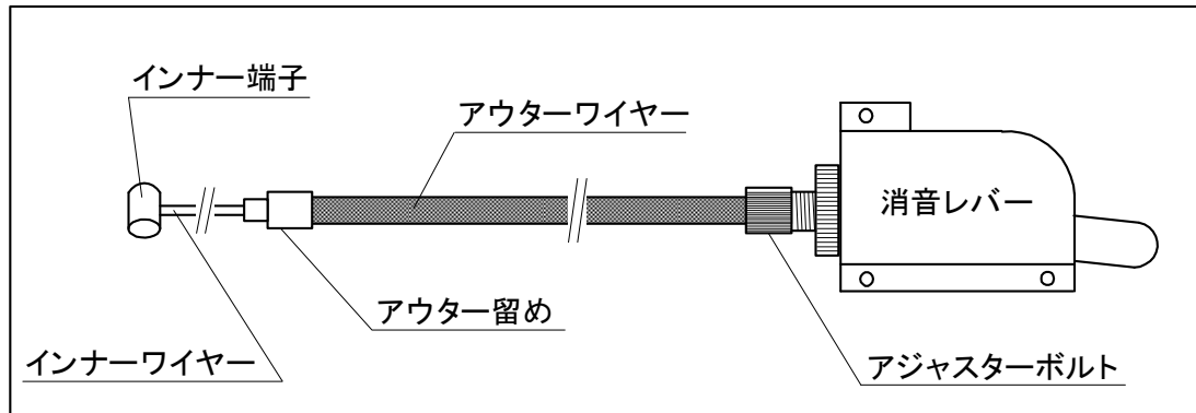
図 4. 6 - 1 消音レバー全体図
