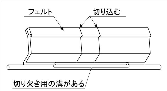
図 4. 2 - 2 中音部の加工方法
