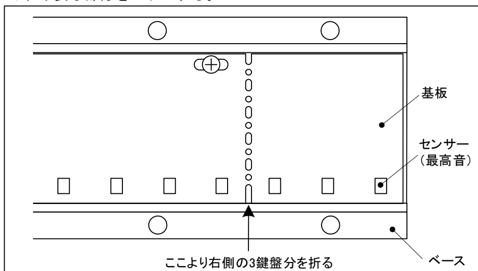
図4.4-10 85鍵盤ピアノへの取り付け
