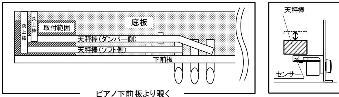
図 4. 5 - 5 センサー部の逆付け
