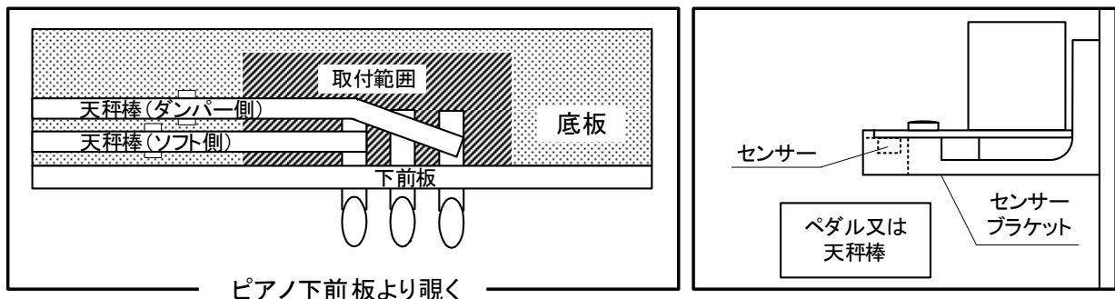
図4. 5 - 1 ペダルセンサーの取り付け
