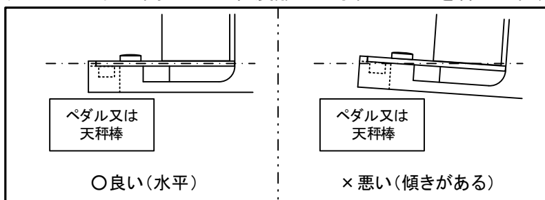
図 4. 5 - 4 センサー部の取り付け状態
