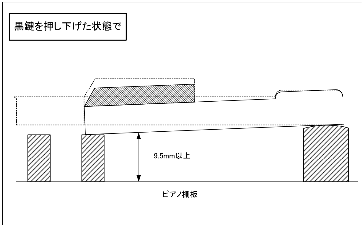
図 4. 4 - 1 鍵盤下の寸法
