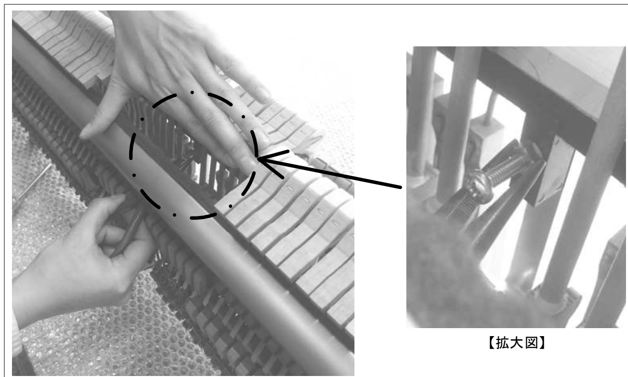
図 4. 3 - 9 M4ナットの締め方
