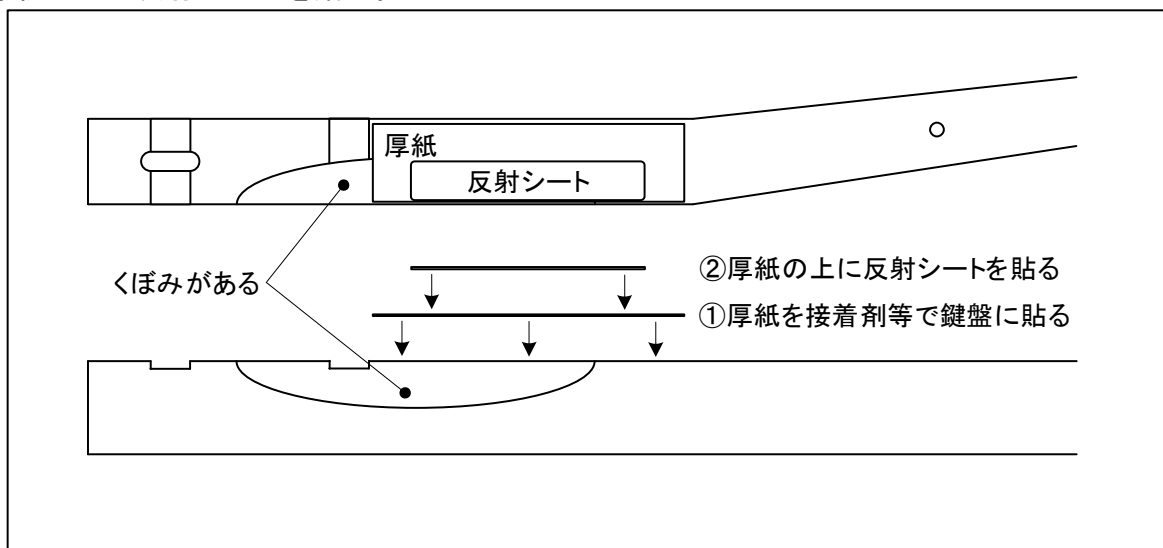
図4.4-9 くぼみがある鍵盤への反射シートの貼り付け
