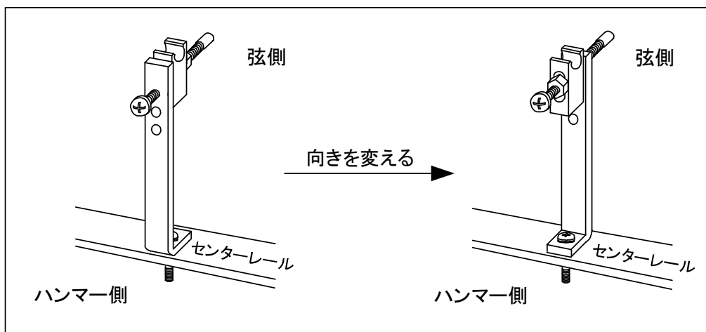
図 4. 3 - 1 1 サポート金具の向きを変える
