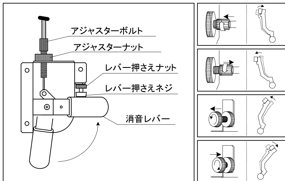
図 4. 8 - 1 ハンマーを止める位置の調整
