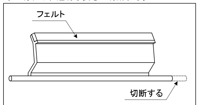
図 4. 2 - 3 高音部の加工方法
