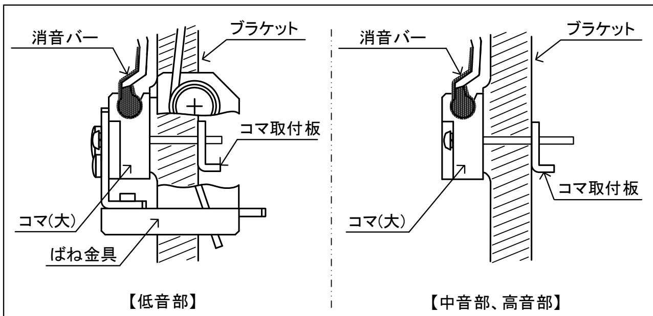
図 4. 3 - 3 ブラケットに取付穴がない場合の取り付け
