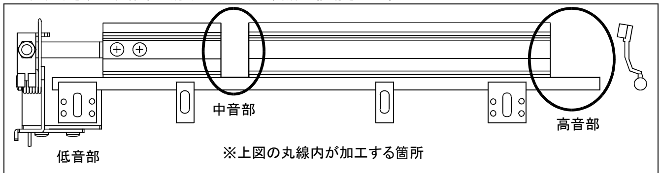
図 4. 2 - 1 消音バーの加工箇所
