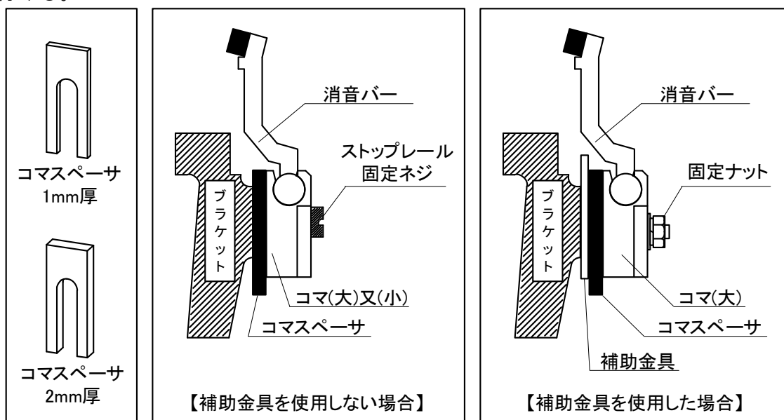
図 4. 3 - 10 コマスペーサによる調整
