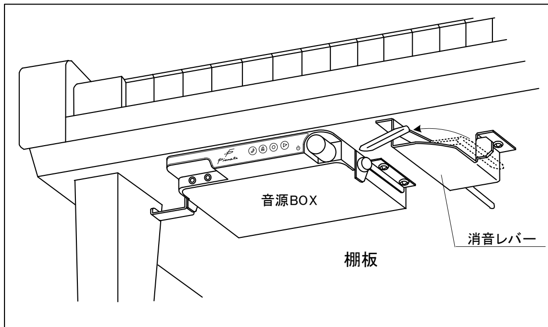
図 4. 7 - 1 音源BOXの取り付け位置
