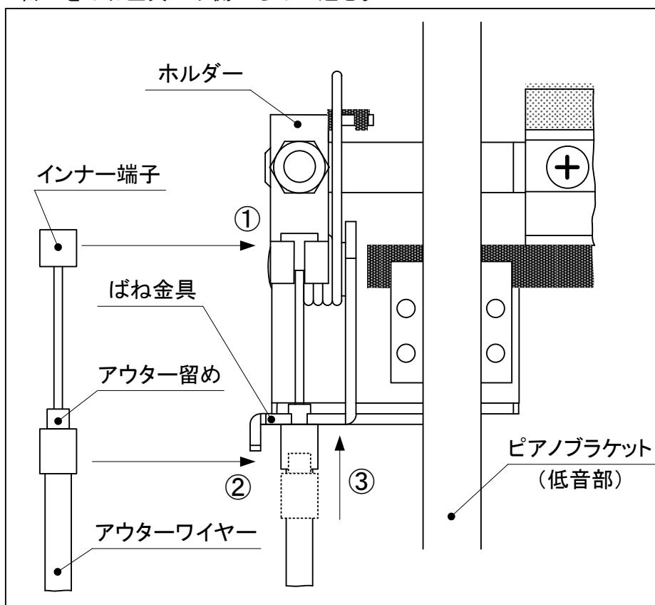
図 4. 6 - 3 ワイヤーの掛け方
