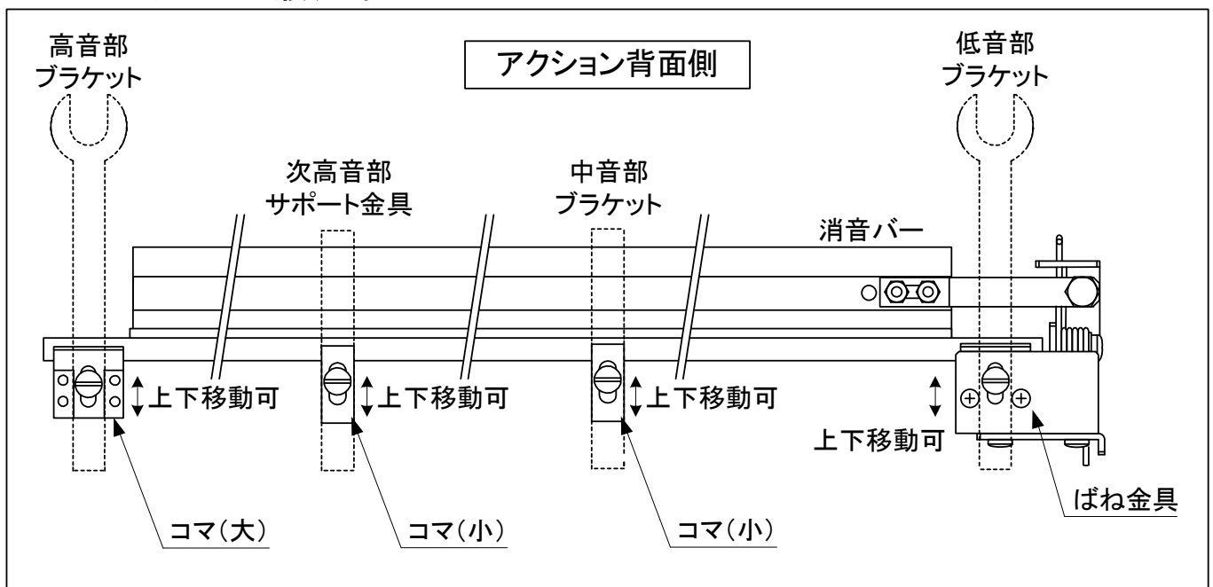
図 4. 3 - 2 消音バーの取り付け
