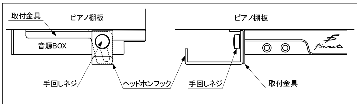
図 4. 7 - 2 ヘッドホンフックの取り付け
