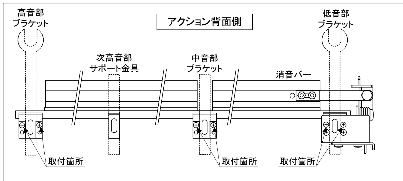
図 4. 3 - 4 取付箇所
