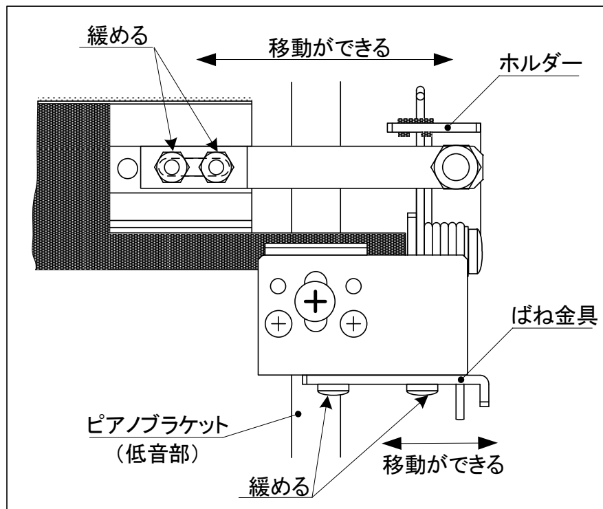
図 4. 3 - 1 2 ホルダーとばね金具の移動
