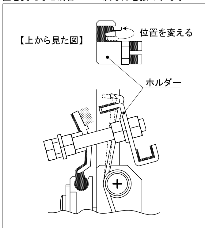
図 4. 3 - 1 3 消音バーの戻りを強くする
