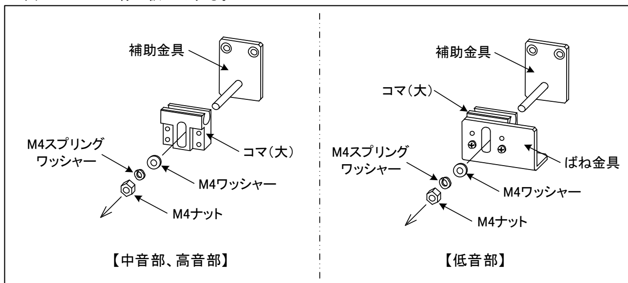
図4.3-5 補助金具の仮止め
