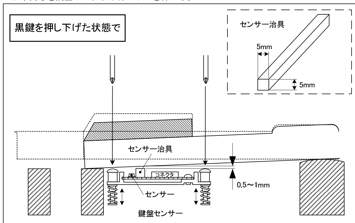
図4.4-6 鍵盤センサー取り付け高さ調整
