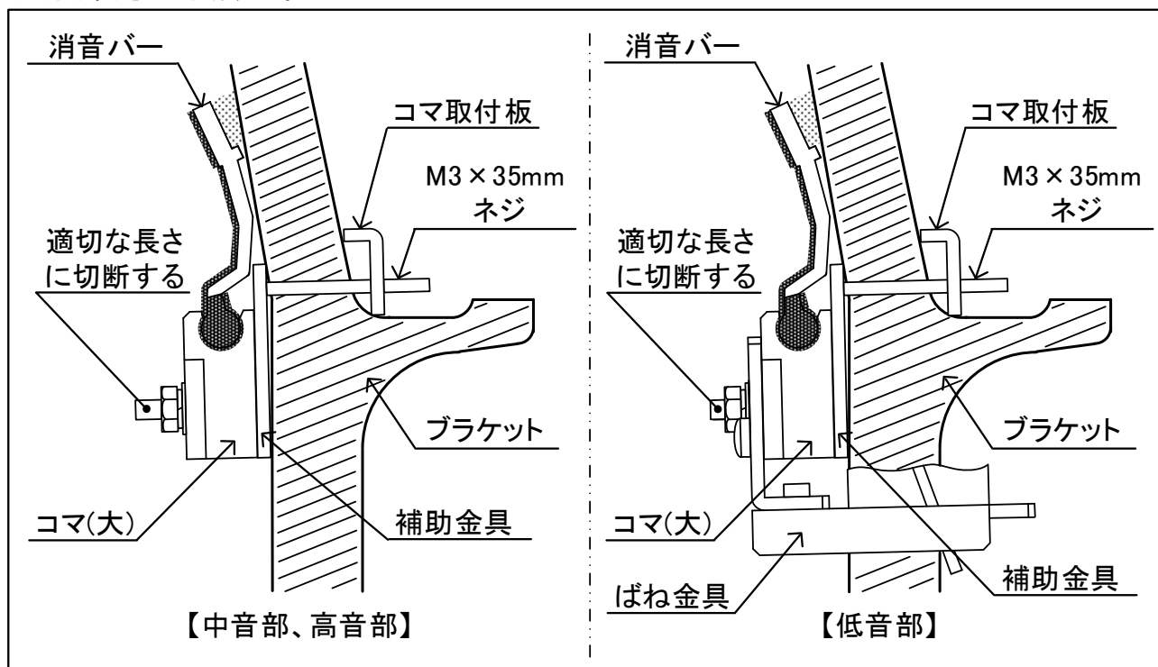
図4.3-6 低音部、中音部、高音部の取り付け
