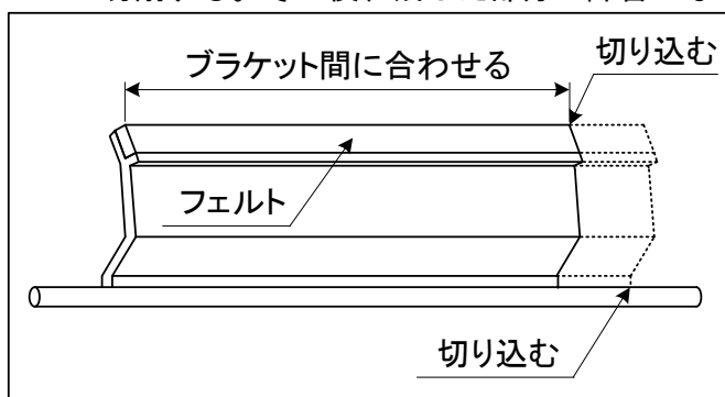
図 4. 2 - 3 高音部の加工方法
