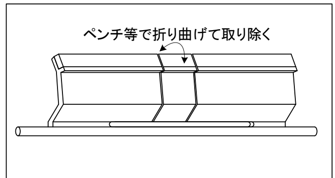
図 4. 2 - 2 中音部の加工方法
