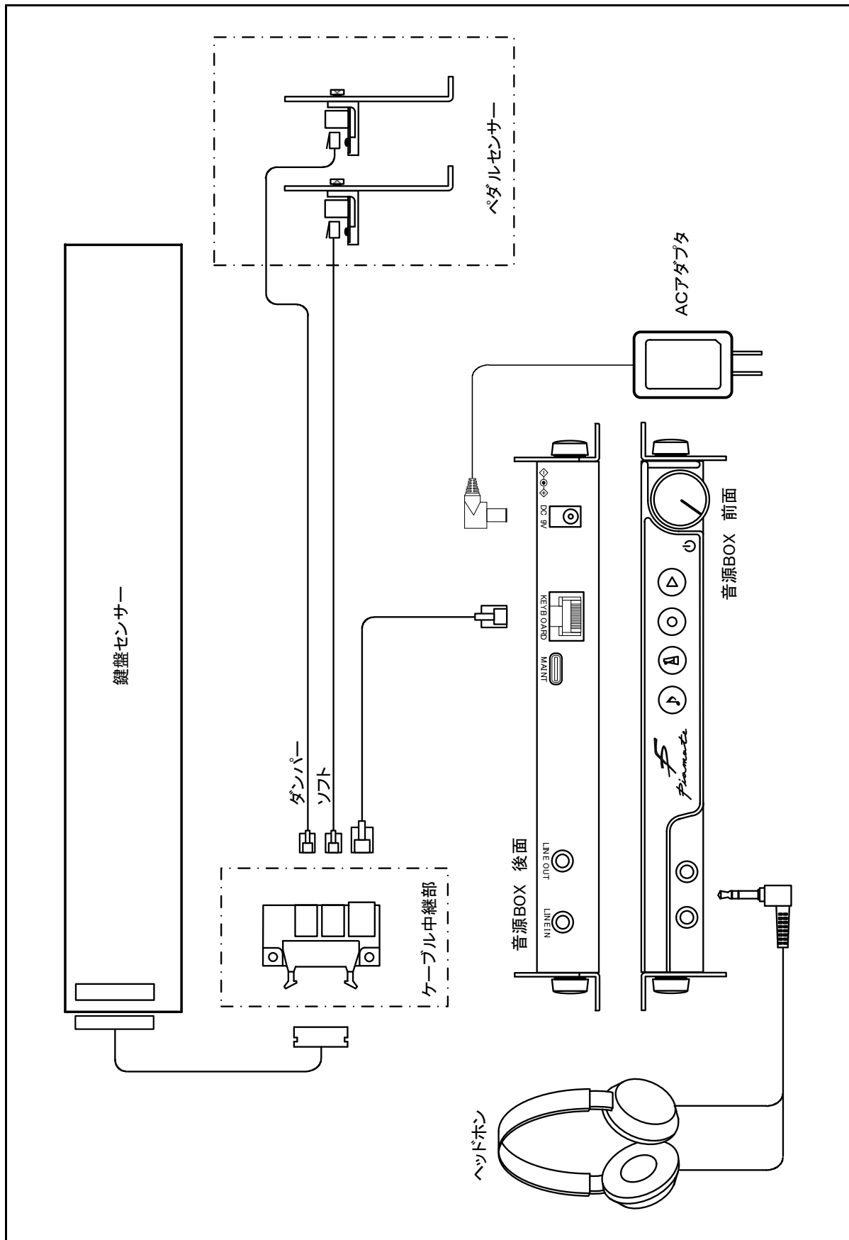
Piamate接続図
