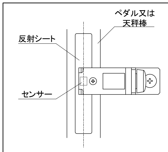
図 4. 5 - 3 反射シートの貼り付け
