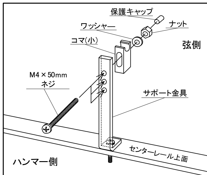
図 4. 3 - 7 サポート金具での消音バーの取り付け
