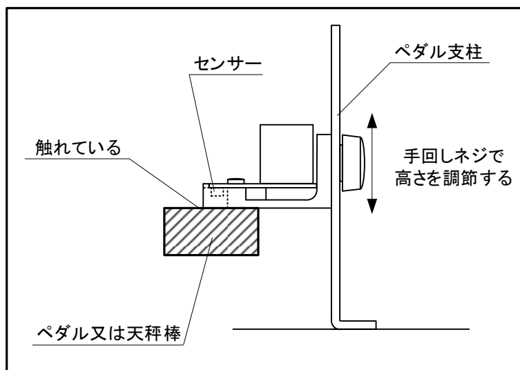
図4. 5 - 2 センサー部の高さ調整
